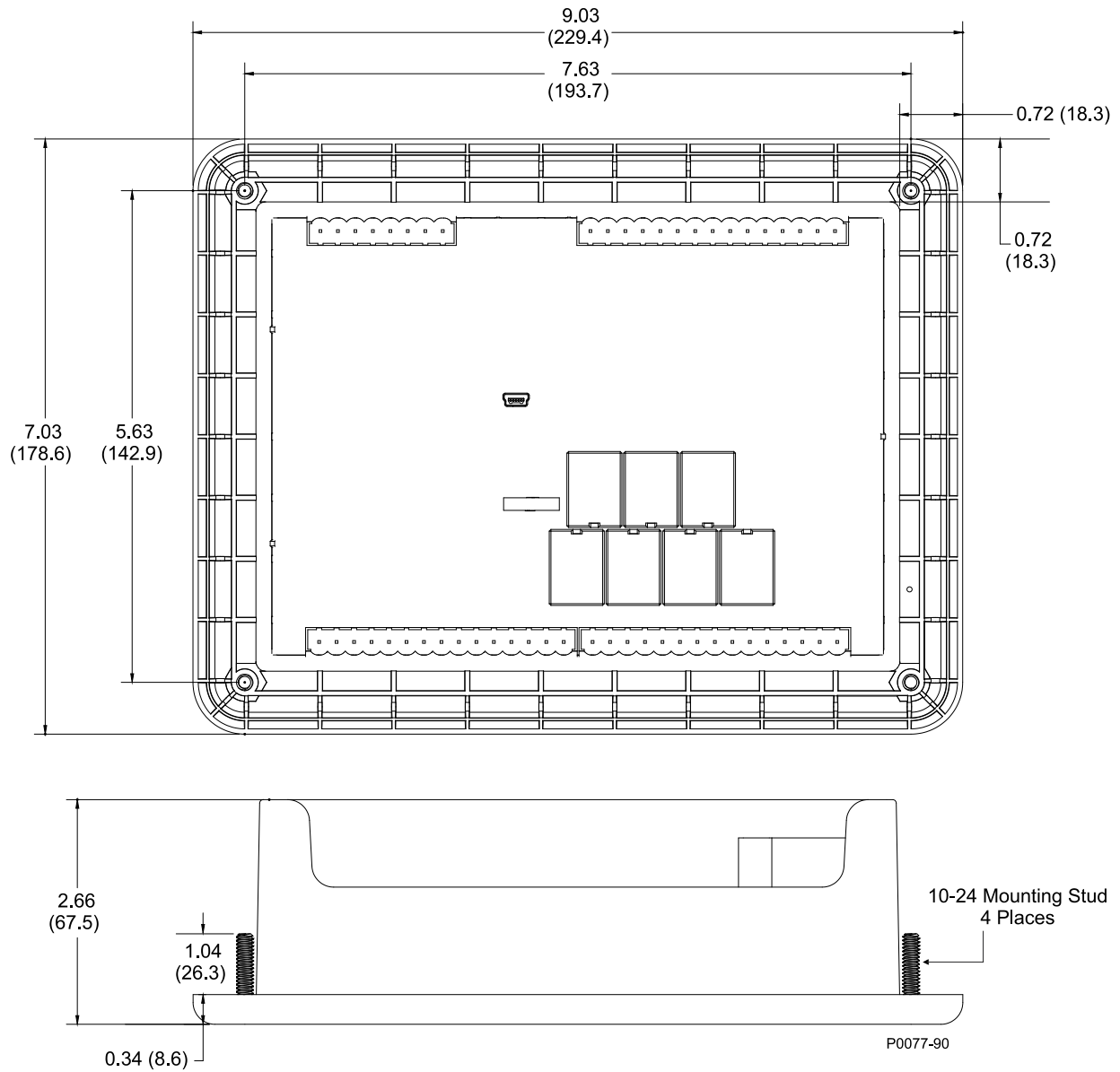
Figura 1-2. Dimensiones Generales
