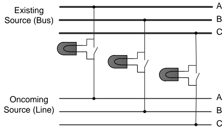
Fig. 2a Dark Lamps
