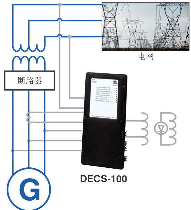
图 1 - DECS-100典型应用接线图
